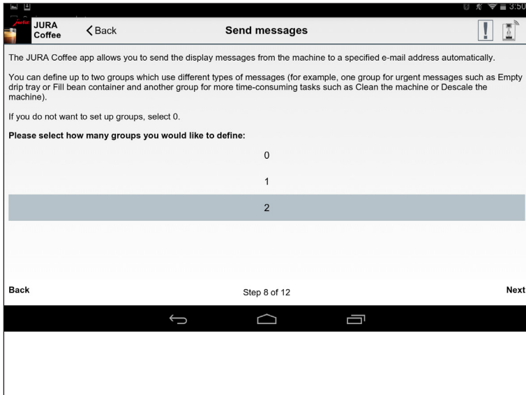
Fig. 47: Sending messages
